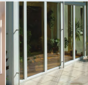
Puertas Osciloparalela
